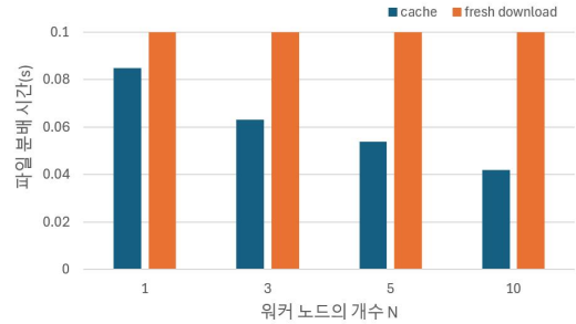
그림 1 워커 노드의 개수에 따른 파일 분배 시간
