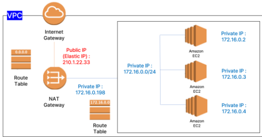
(그림 1) AWS 기반의 망분리 인프라 제안
