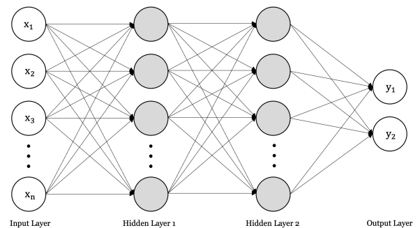
그림 1. DNN architecture
