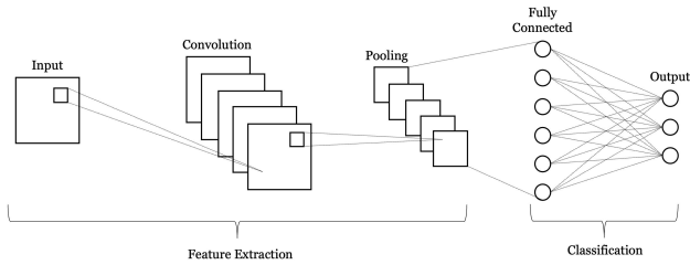
그림 2. CNN architecture
